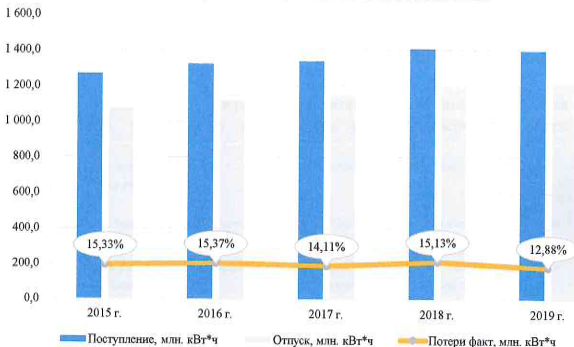
Баланс электрической энергии за 2015-2019 гг. млн. кВт. час.
